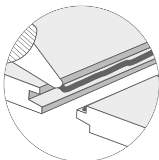
Sklížení profilu pero-drážka
