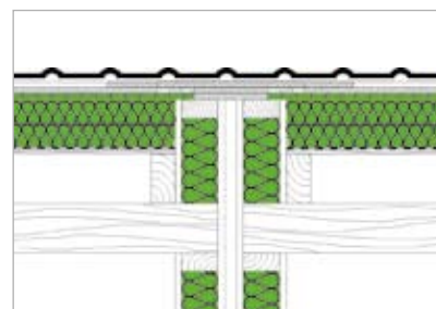
Napojení dělicí stěny mezi domy u řadového domu (se stojatým štítem)
