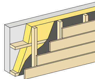
Obr. 1 - Nosná konstrukce tvořená vodorovnými a svislými nosníky
