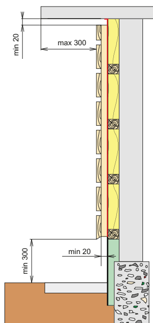
Schéma minimálních a maximálních odstupů
