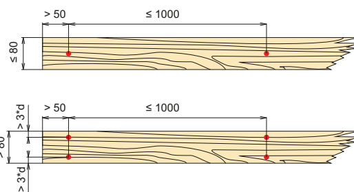
Schéma minimálních a maximálních vzdáleností spojovacího materiálu u prken
