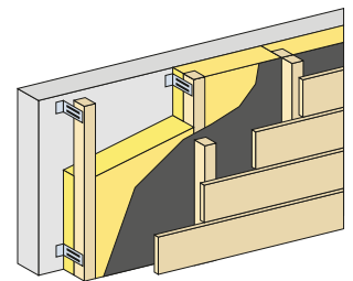
Obr. 3 - Nosná konstrukce tvořená svislými nosníky na ocelových úhelnících
